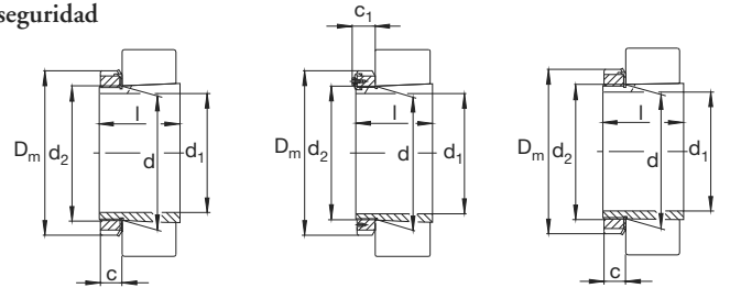
Cono 1:12 Chapa de seguridad MB, MBL Cono 1:12 Grapa de seguridad MS30 Cono 1:30 (H240) Chapa de seguridad MBL
