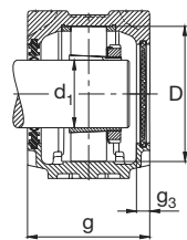
Obtención de doble labio DH Tapa DKV
