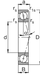
B719C, B70C Angulo de contacto \alpha = 15^\circ
