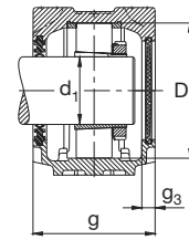
Obturación de doble labio DH Tapa DKV
