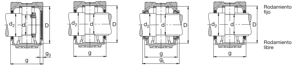
Obturator de doble labio DH Tapa DKV Obturator de doble labio DH Anillo de laberinto TSV Obturator de filtro FSV
