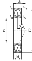
B719E, B70E Angulo de contacto \alpha = 25^\circ
