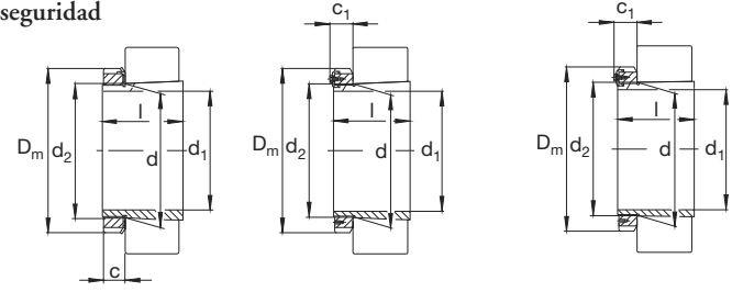
Cono 1:12 Chapa de seguridad MB Cono 1:12 Grapa de seguridad MS30, MS31 Cono 1:30 (H240, H241)
