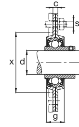
FBB2 combinado con 562
