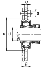
FBB2 combinado con 362
