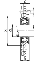
FBB2 combinado con 762..2RSR
