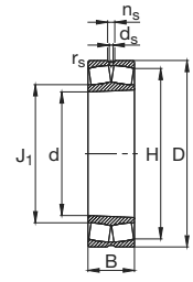
K Agujero cónico (cono 1:12)
