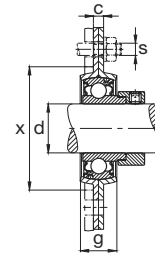
FBB2 combinado con 162
