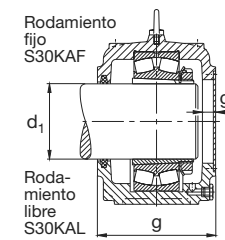
Ejecución A desde S3044K
